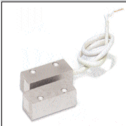
C401 : Contact de porte et fenêtre magnétique aluminium en applique, sortie 4 fils. Dimensions 17x10x43mm.
