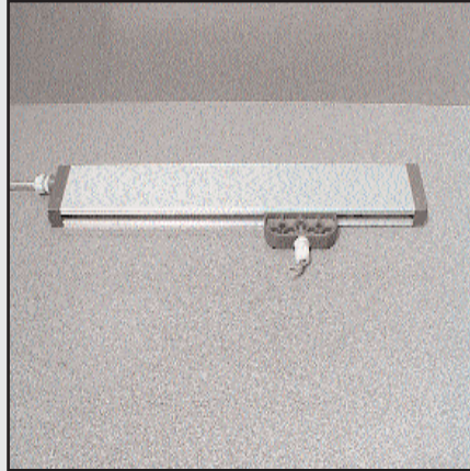
ALCOMA: rail pour tranche de sécurité (palpeur) embarquée sur portail coulissant pour tous types de palpeurs (5 conducteurs) recoupables. Nous préparons le rail à la longueur désirée, sur commande.
