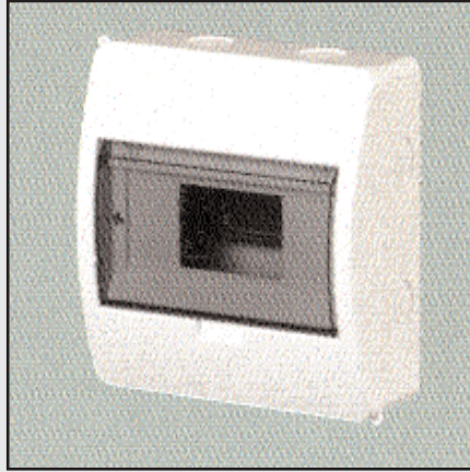
066300IP30D : Coffret 8 modules , IP30D , 195x195x90 , équipé avec porte transparente et terminal N+PE.
