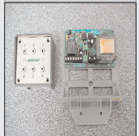
IDTAST : Clavier à codes filaire numérique BENINCA avec son récepteur.
