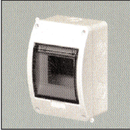
066100IP30D : Coffret 5 modules , IP30D , 156x116x93 , équipé avec porte transparente et terminal N+PE.
