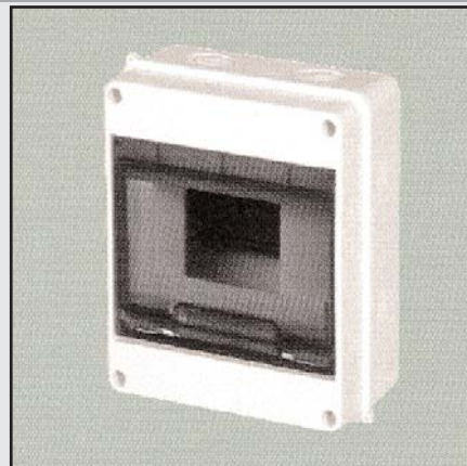
061600IP55 : Coffret 9 modules , IP55 , 197x197x95 , équipé avec porte transparente et terminal N+PE.
