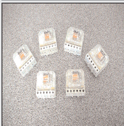
Télérupteurs 10A , série 26 .REF : 2601 unipolaire 24vac , 2601 unipolaire 220vac , 2602 bipolaire 24vac , 2602220 bipolaire 220v , 2603 inverseur 24vac , 2603220 inverseur 220vac , 2608 séquentiel 24vac , 2608220 séquentiel 220vac ,260212 12v.
