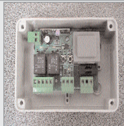
2022 : Kit de commande radio pour 2 circuits d'éclairage, 2 relais de 7 A. 3 programmations possibles : impulsionnel, têlêrupteur et têlêrupteur temporisê de 0 à 64 mn. Entrêes boutons pousseirs. P46. Il s'agit d'un contact sec.
