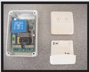
KCTR29LBEE : gestion d'éclairage par bouton poussoir radio , 2 circuits 2x1000w.
