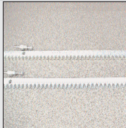
3012V : crémaillère en acier galvanisé livrée avec supports à visser. Module 4. Vendue au mètre.
