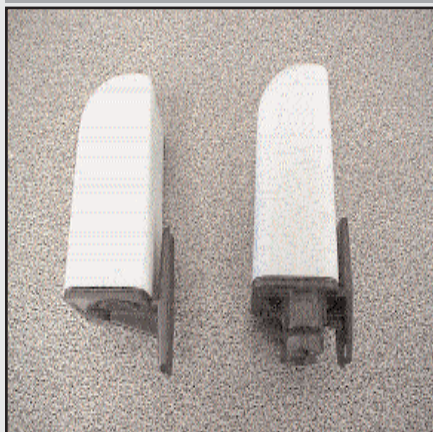
C01 : Relais crépusculaire 220v fixation sur poteau non réglable 10 lux 1200w . C01A : Relais crépusculaire 220v fixation sur poteau sensibilité réglable de 2 à 80 lux 2700w .
