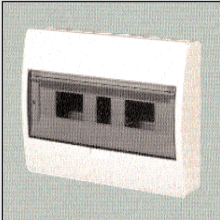
066900IP30D : Coffret 24 modules , IP30D , 406x303x98 , équipé avec porte transparente et terminal N+PE.
