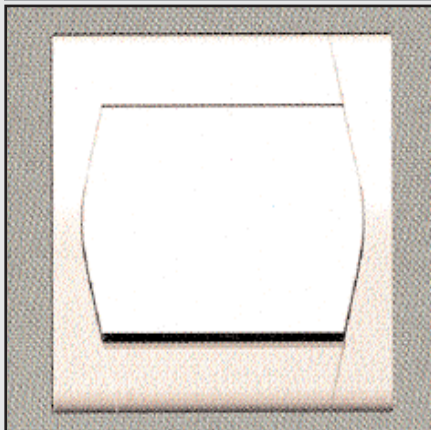
85100 : Interrupteur simple IP20 10A/250V blanc à encastrer. Gamme FESTA.
