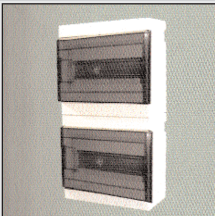
060500IP20 : Coffret 16 modules , IP20 , 340x170x97 , équipé avec porte transparente et terminal N+PE.
