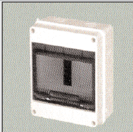
061800IP55 : Coffret 7 modules , IP55 , 161x174x93 , équipé avec porte transparente et terminal N+PE.
