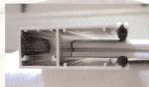
Toutes nos coussins comportent joints de frottement et joint brosse d'étanchéité.
