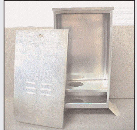
ARCG : coffret en acier galvanisé à clés Dimensions : L280xH700xP170 mm L = largeur H = hauteur P = profondeur Livré support à sceller ou à boulonner . Idéal pour l'installation d'un coffret de gestion pour moteur coulissant en copropriété et usine .
