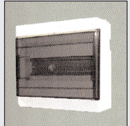
060300IP20 : Coffret 12 modules , IP20 , 170x245x97 , équipé avec porte transparente et terminal N+PE.
