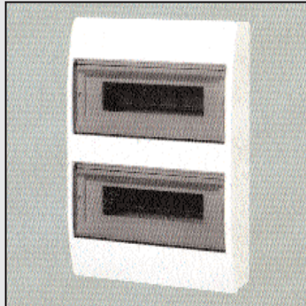
067000IP30D : Coffret 36 modules , IP30D , 784x410x98 , équipé avec porte transparente et terminal N+PE.
