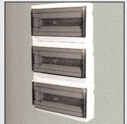
060900IP20 : Coffret 36 modules , IP20 , 510x245x97 , équipé avec porte transparente et terminal N+PE.
