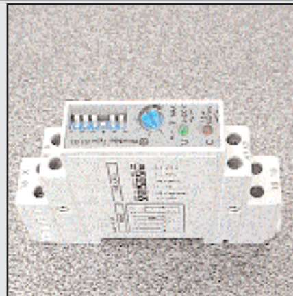
8101 : Temporisateur électronique multi-fonctions et multitensions modulaire , toutes tensions et tous types de fonctionnements .
