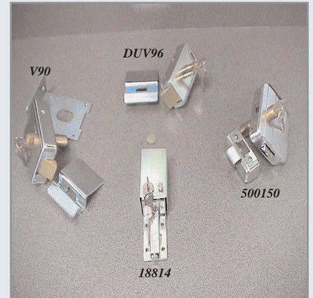
Serrures électriques : DUV96 : serrure élec verticale à pêne basculant 12v V90 : serrure élec verticale à pêne basculant 12v 18814 : ser élec verticale pêne rentrant 24v ou 220v 500150 : serrure élec standard à pêne rentrant 12v
