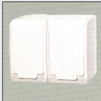
32202 : Prise de courant double , IP44 16A/250V , blanc capôt blanc ,avec éclips de protection enfant , en saillie.Gamme HERMES.
