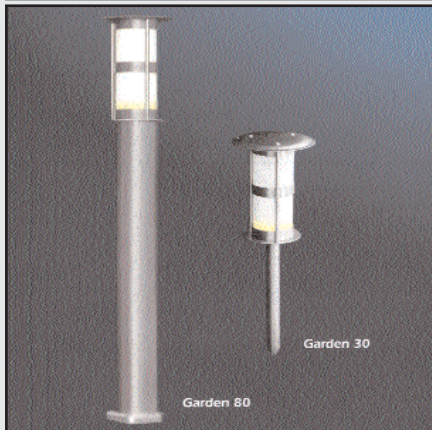
GARDEN30: Lampe inox 60w set à 2 pièces, alim 12v.
