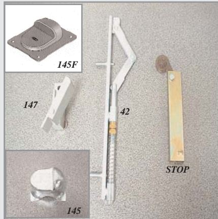
145 : Butée au sol portail fermé à sceller . 145F : Butée au sol portail fermé à visser . 42 : bloqueur à tige. STOP : bloqueur feuillure. 147 : bloqueur à bascule.
