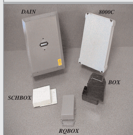
Coffrets vides en ABS : L : largeur , H : hauteur , P : profondeur DAIN : coffret à vis dim L220xH270xP110 8000C : coffret à vis dim L170xH235xP90 SCHBOX : coffret dim L100xH82xP30 RQBOX : coffret dim L110xH65xP30 BOX : coffret pour petite électronique
