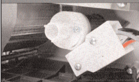
Fin de course électromécanique incorporée actionnés par un bouton facilement réglable
