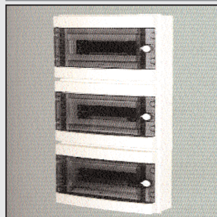
063400IP55 : Coffret 57 modules , IP55 , 788x410x150 , équipé avec porte transparente et terminal N+PE.
