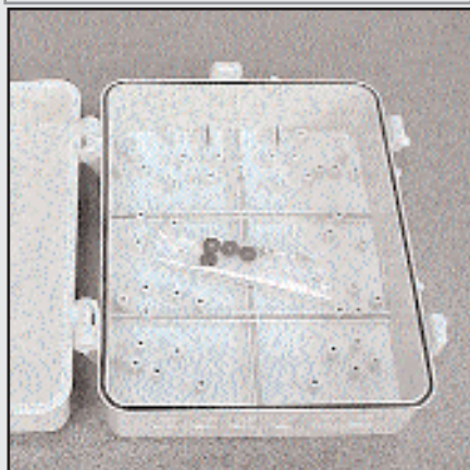
ASC31 : coffret à charnières en ABS Dimensions : L180xH230xP90 mm angles en arrondi L = largeur H = hauteur P = profondeur
