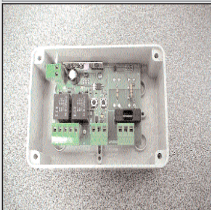
I022 : Système de pilotage de mise en route et arrêt de l'alarme avec en option une télécommande. Intègre la possibilité d'extension avec un nombre illimité de détecteurs radio RHB .
