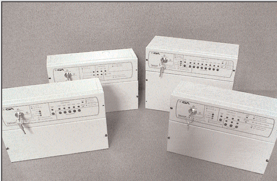
PROTEC3 : Centrales d'alarme filaires professionnelles en ABS : 2 zones. Zones sélectionnables en façade. Mise en service et arrêt par clé personnalisée sur panneau frontal.
