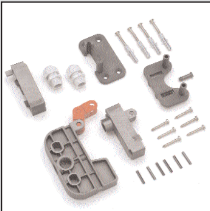
AKSKIMOF2: set montage au détail pour ALCOMA (livré dans ALCOMA).
