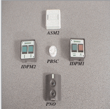
Boutons poussoirs : PB5C : bouton poussoir saillie ASM2 : bouton poussoir en saillie 2 contacts IDPM2 : bouton poussoir en saillie 2 contacts IDPM1 : bouton poussoir en saillie 2 contacts PNO : bouton poussoir en saillie 2 contacts VOIR RUBRIQUE ORGANES DE COMMANDE
