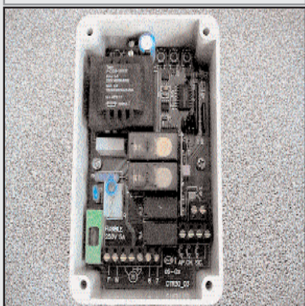
CTR30 : Coffret de commande 1 moteur 220V pour rideau métallique avec récepteur intégré. Réglage force, temps de travail, pause et accessoires de sécurité. Contact montée , contact descente , contact montée/descente , 12V pour accessoires , réglage de puissance possible en option , bornier antenne et de nombreux pas de programmes .Coffret de gestion de très petites dimensions . EX : Rideau
