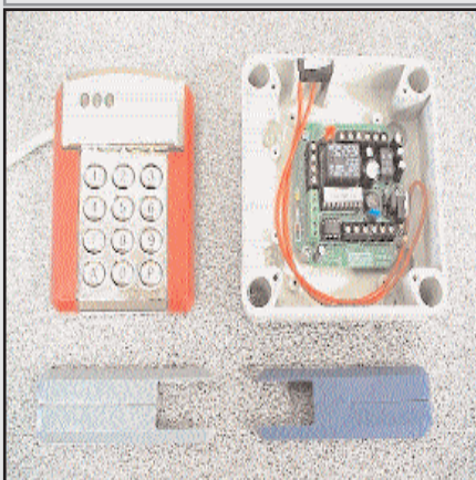
SUN : Clavier à codes autonome, 2 relais, 250 codes utilisateurs. IP67 totalement anti vandal, ultra plat. Electronique déportée . Polyvalent : contrôle d'accès, alarme, automatisme. Le Clavier sup SUNC .
