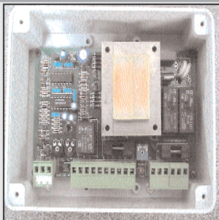
TT120 : Petite platine électronique 1 moteur 220V avec fin de course. Taille réduite à insérer dans moteur. Contact fin de course ouverture et fermeture, feu de signalisation, alim 24V, stop arrêt urgence, tranche de sécurité, photocellules. Réglage puissance moteur, temps de pause et travail. Programmmations en automatique et pas à pas. LIVRE SANS LE COFFRET.
