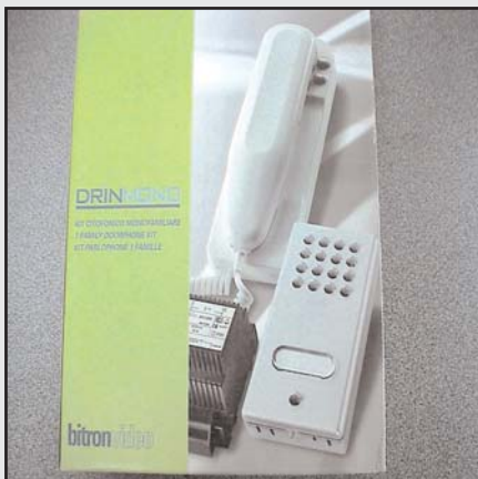
DRIN : Interphone filaire (5 fils), 1 poste, plaque de rue en applique extra plate aluminium, avec 2 boutons pour ouverture du portail et gache sur le combiné intérieur. Très bonne phonie jusqu'à 400mètres de distance.
