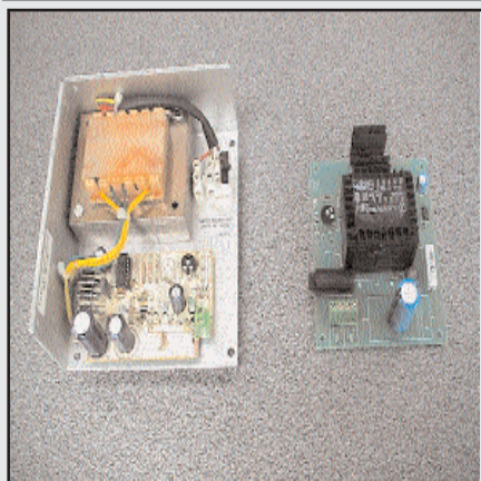
AEAL05 : Alimentation 117/240v, sortie 12vdc 0.5A. AL3A : Alimentation 117/240v, sortie 12vdc 3A.
