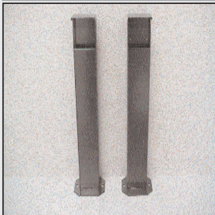
P41C : Colonne acier tôle pliée hauteur 500mm pour cellules saillie P41 .
