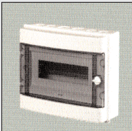
062000IP55 : Coffret 13 modules , IP55 , 213x302x116 , équipé avec porte transparente et terminal N+PE.
