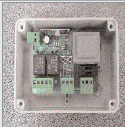
2022 : Kit de commande radio pour 2 circuits d'éclairage, 2 relais de 7 A. 3 programmations possibles : impulsif, télérupteur et télérupteur temporisé de 0 à 64 mn. Entrées boutons poussoirs. P46. Il s'agit d'un contact sec.
