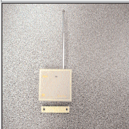
RCMS1 : Contact de porte et fenêtre radio 9Vcc. Fonctionne avec coffret de gestion I022 ..
