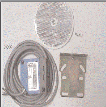
FQ06 : Cellules reflex non étanches 220vac/dc portée de 7 mètres. WAB : réflecteur rond de la cellule.
