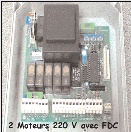
STU3 : Coffret de commande universel pour 2 moteurs en 220V avec ou sans fin de course ou bien 2 coulissants avec leurs fins de course respectifs . Toutes les options possibles sont présentes comme dans la 8000S .Réglage puissance moteur, temps de travail, de pause, décalage des vantaux. Programmations en automatique ou en pas à pas ...
