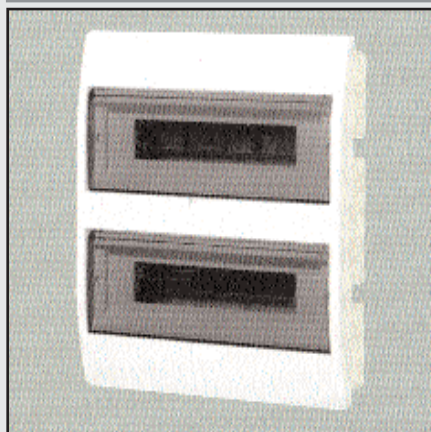
065510IP30D : Coffret 24 modules , IP30D , 406x303x103 , équipé avec porte transparente et terminal N+PE.A encastrer.
