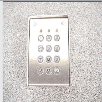
SU2SAB : Clavier à codes en saillie dans son boîtier de protection en acier 2 relais NO/NF 12/24V pour mise en route et arrêt du système d'alarme.Témoins lumineux par leds .Rétroéclairage .
