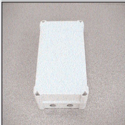
8000C : coffret à visser en ABS Dimensions : L170xH235xP90 mm L = largeur H = hauteur P = profondeur
