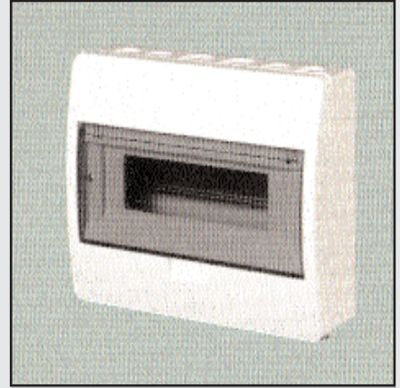
066500IP30D : Coffret 12 modules , IP30D , 212x303x98 , équipé avec porte transparente et terminal N+PE.
