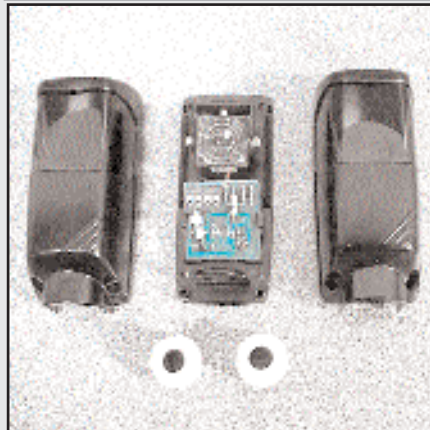
CDR842A : Cellules anti vandalisme dans boîtier aluminium. Longue portée, orientables à 180°. Portée maxi 30 mètres.
