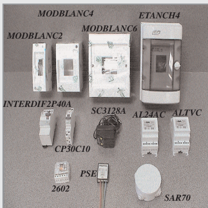
MODBLANC4 , ETANCH4 MODBLANC2 , MODBLANC6 INTERDIF2P40A : interruptif différentiel 2 pôles 40A CP30C10 : disjoncteur 10 A SC3128A : alim universelle 12v DC AL24AC/ALTVC : alim 24vac et alim 12vdc 250mA 2602 : télérupteur 24vac 2x10A PSE : Parafoudre à gaz SAR70
