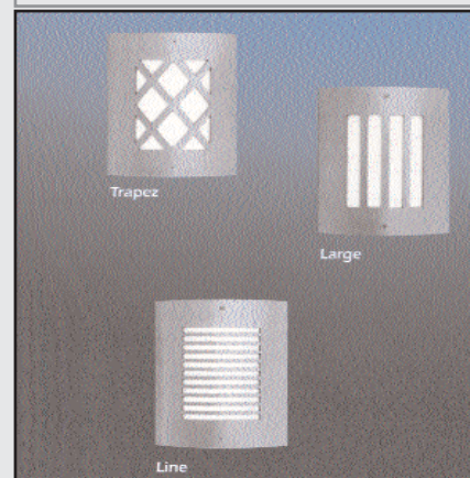
TRAPEZS: Lampe murale inox 60w. Avec détecteur 180°/15m, orientable 90°. LARGES: Lampe murale inox 60w. Avec détecteur 180°/15m, orientable 90°. LINES: Lampe murale inox 60w. Avec détecteur 180°/15m, orientable 90°.
