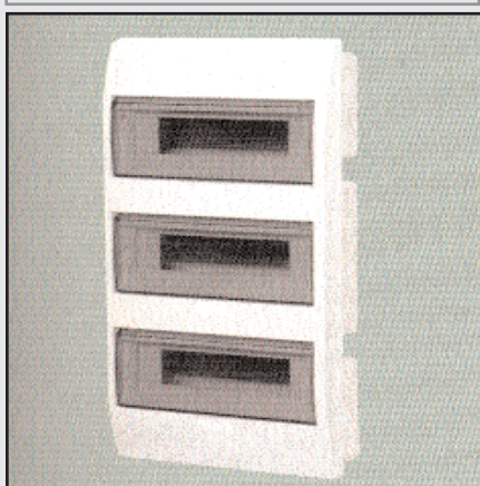
065710IP30D : Coffret 36 modules , IP30D , 550x303x105 , équipé avec porte transparente et terminal N+PE.A encastrer.
