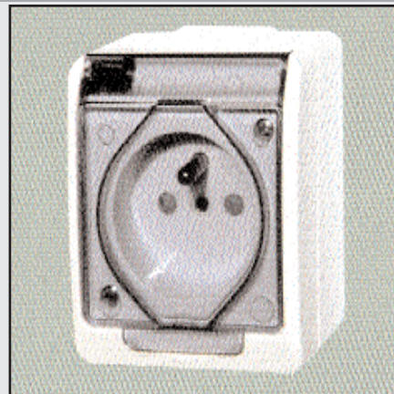
32101 : Prise de courant simple , IP44 16A/250V , bi-color capôt fumé ,avec éclips de protection enfant , en saillie.Gamme HERMES.
