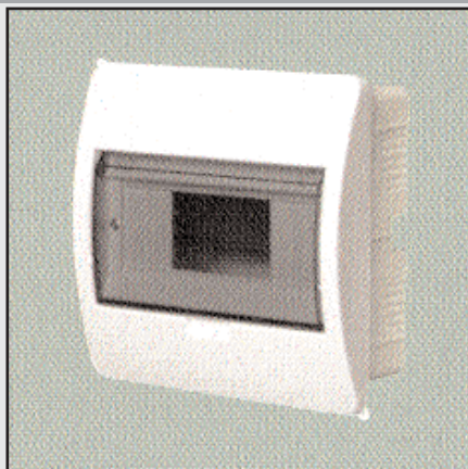
064510IP30D : Coffret 8 modules , IP30D , 195x195x105 , équipé avec porte transparente et terminal N+PE.A encastrer.
