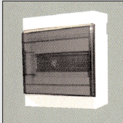
060200IP20 : Coffret 6 modules , IP20 , 170x170x97 , équipé avec porte transparente .
